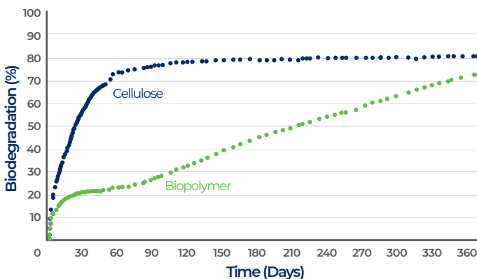
Curva ejemplo de biodegradación de un biopolímero comparado con el control positivo estándar. Fuente: aut. SAMCA.
